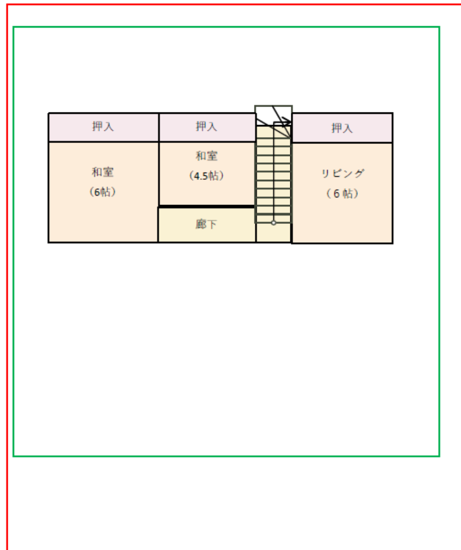
2F間取り
