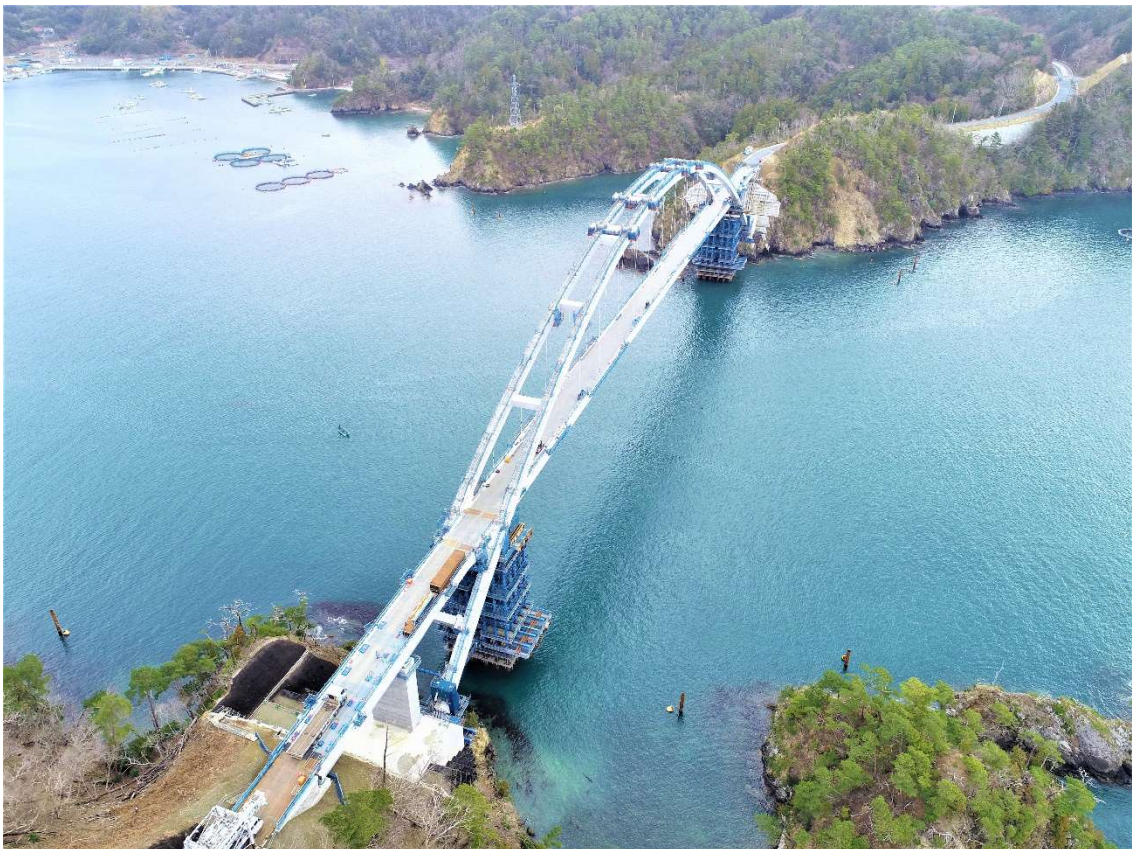
(出島架橋現地の状況 (南西側から))
